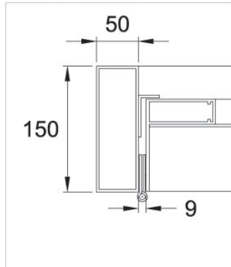
Jamb detail
